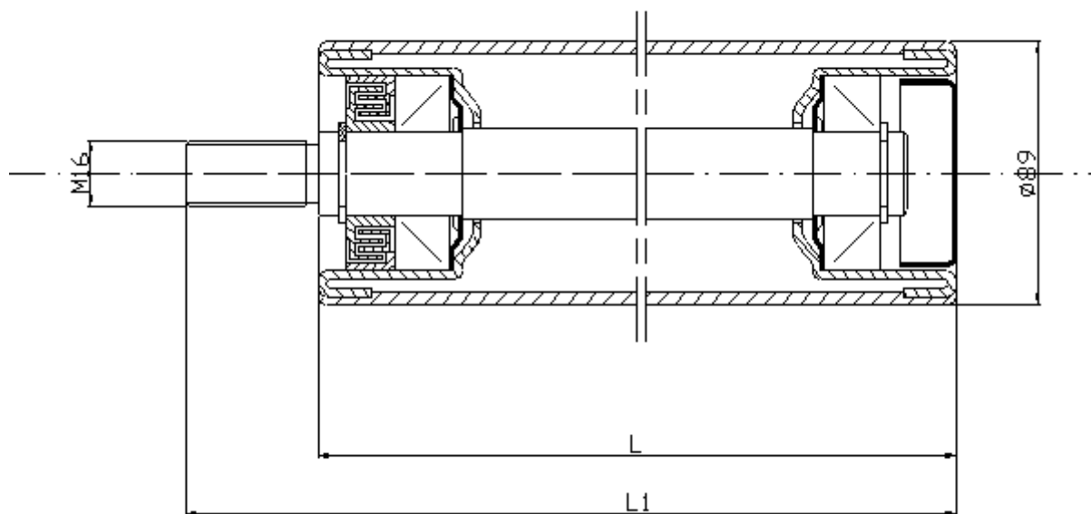
krążnik kierunkowy \varnothing 89/\varnothing 108/\varnothing 20 -L
