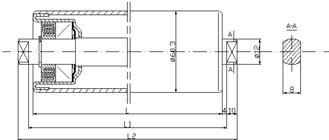
krążnik kierunkowy \varnothing 60,3/\varnothing 20-L
