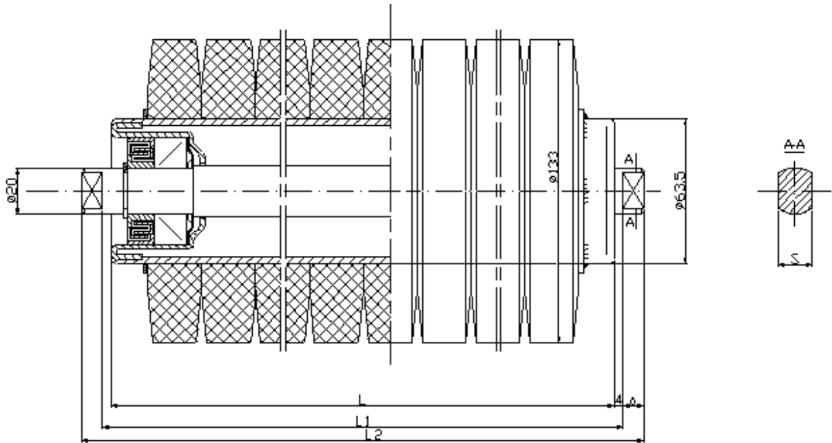
krążnik pierścieniowy \varnothing 133/\varnothing 20-L
