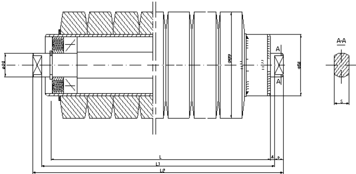
krążnik pierścieniowy \varnothing 89/\varnothing 20-L
