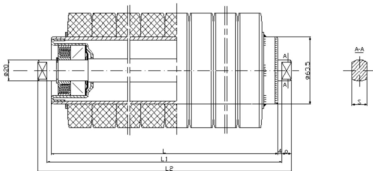
krążnik pierścieniowy \varnothing 108/\varnothing 20-L
